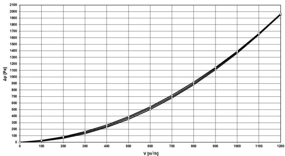
Рис. 16: Диаграмма падения давления
