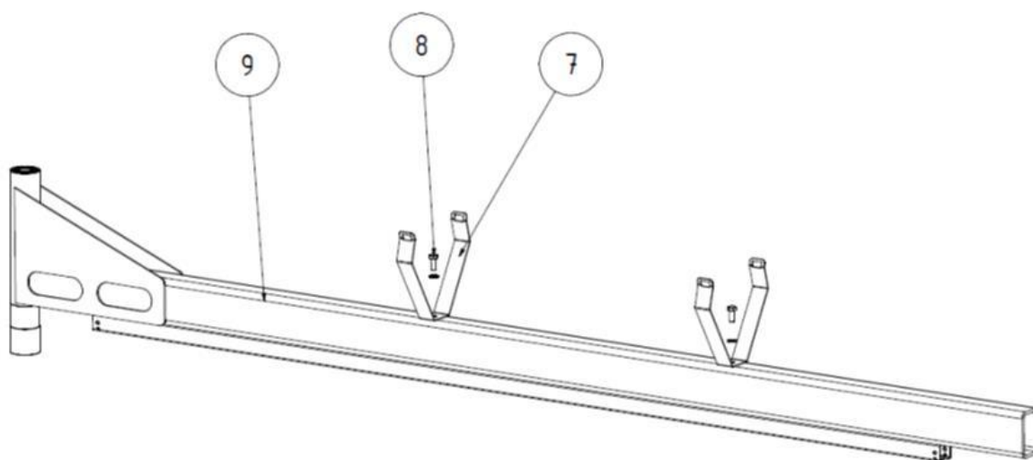
Рис. 5: Узел крепления трубы и крепление вытяжного рукава
