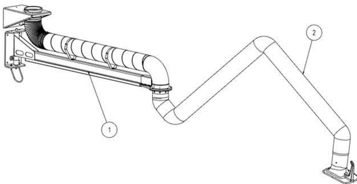
Рис. 1: Вытяжной рукав с поворотной консолью
