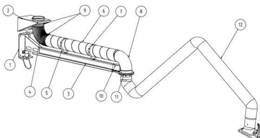
Рис. 3: Консоль с вытяжным рукавом
