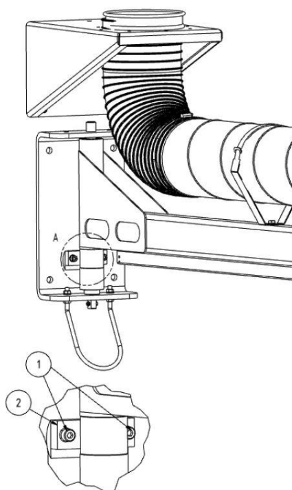
Рис. 11: Тормоз консоли
