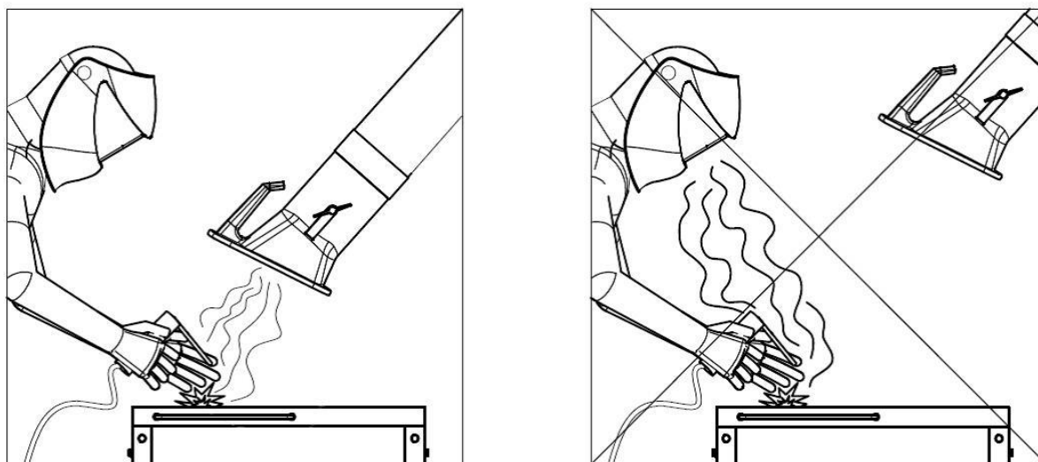
Рис. 15: Установка вытяжного колпака
